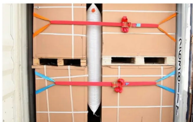
Systemy do mocowania w kontenerach Block-Load 8000
