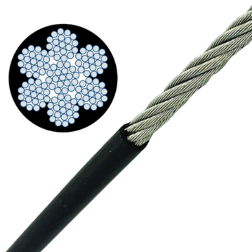
Liny stalowe PVC Black
