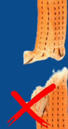
Pęknięcie / przecięcie taśmy Nacięcia, rozdarcia, ubytki włókien, które są głębokie, długie lub obejmują kilka nitek nośnych.
